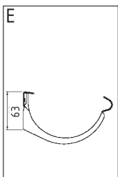
Крюк короткий специальный 125 R2OG125BES
