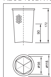
Фильтрующее колено R4OD100S
