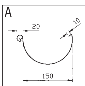
Желоб полукруглый 150 R5OG1502000 R5OG1504000
