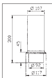
Отвод в колодец 100/300 R4OD100J
