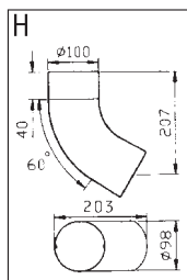
Колено круглое 100 R1OD100N
