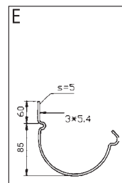
Крюк короткий 125 R2OG125BS
