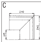
Угол внутренний R1EGCI внешний R1EGCE
