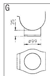
Воротничок от круглого желоба в круглую трубу 150/100 R4OG1501000
