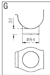
Воротничок от круглого желоба в круглую трубу 125/87 R4OG12587O
