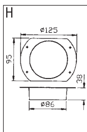
Воротничок от прямоугольного желоба в круглую трубу R4EGE87O
