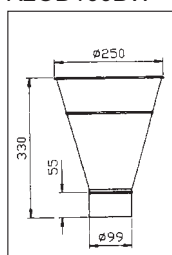
Воронка круглая 100 R4D100W
