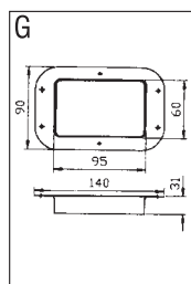
Воротничок от прямоугольного желоба в прямоугольную трубу R4EGEEO
