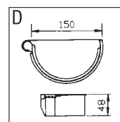
Заглушки желоба 150 R5OG150EP
