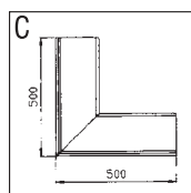
Угол 150 внутренний R1OG150CI90 внешний R1OG150CE90
